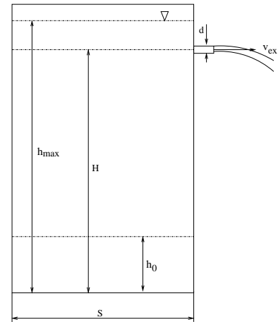
Fig. 1 Serbatoio cilindrico con tubazione di sfioro.
